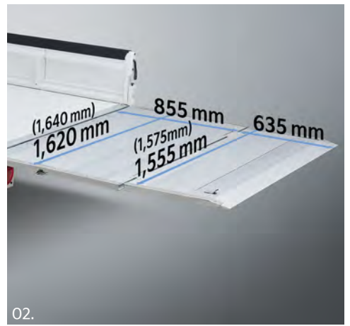
02. 확장형 게이트 규격* ※ ( )는 1.2톤 규격
