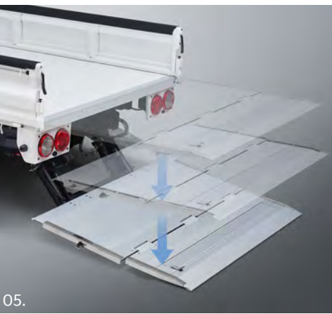
05. 터인형 전동유압식 리프트 시스템*
