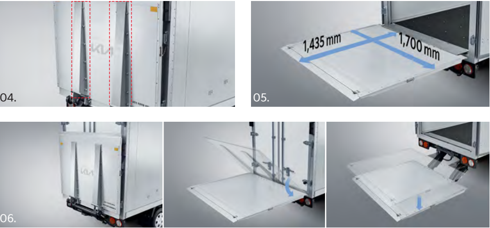
04. 게이트 프레임(받침대)* 06. 게이트 작동순서*
