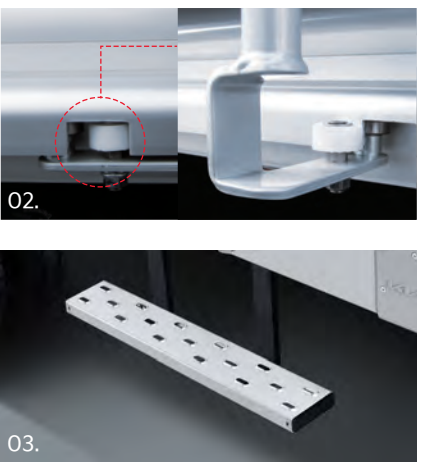
02. 탑 사이드도어 이중베어링 장치 03. 스테인리스 와이드 사이드 스텝
